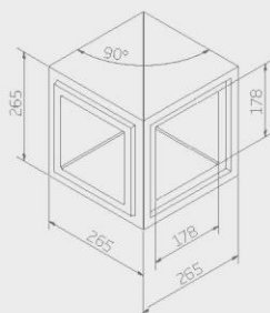
RZUG1 090 830 Lõõrimoodul 18 x 18 90° nurk
