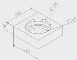
RSNKH SET 010 Lõõrimoodulitest sojussalvesti komplekt II
