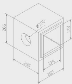
RPUTZ 1M0 722 puhastusava kork Ø100
