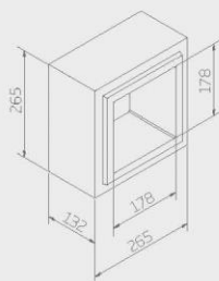
RZUG1 BBN 830 Lõõrimoodul 18 x 18 90° nurk puhastusavaga soone küljel
