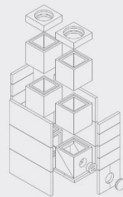
RSNKH SET 010 Lõõrimoodulitest sojussalvesti komplekt II
