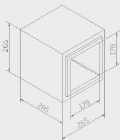
RZUG1 00H 830 Lõõrimoodul 18 x 18 lühike
