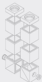
RSNKO SET 010 Lõõrimoodulitest sojussalvesti komplekt I
