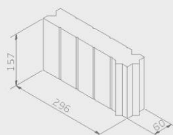
R8632120 005 Quickbrick BR väike
