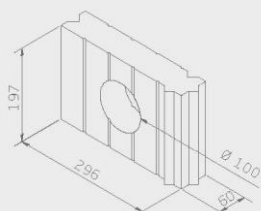
RPUTZ 1M0 722 Puhastusava kork Ø100
